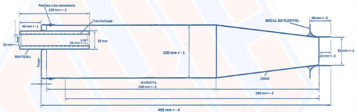
Figura 10 - Desenho Técnico referente ao ARTIGO 37º, PARÁGRAFO 9º
